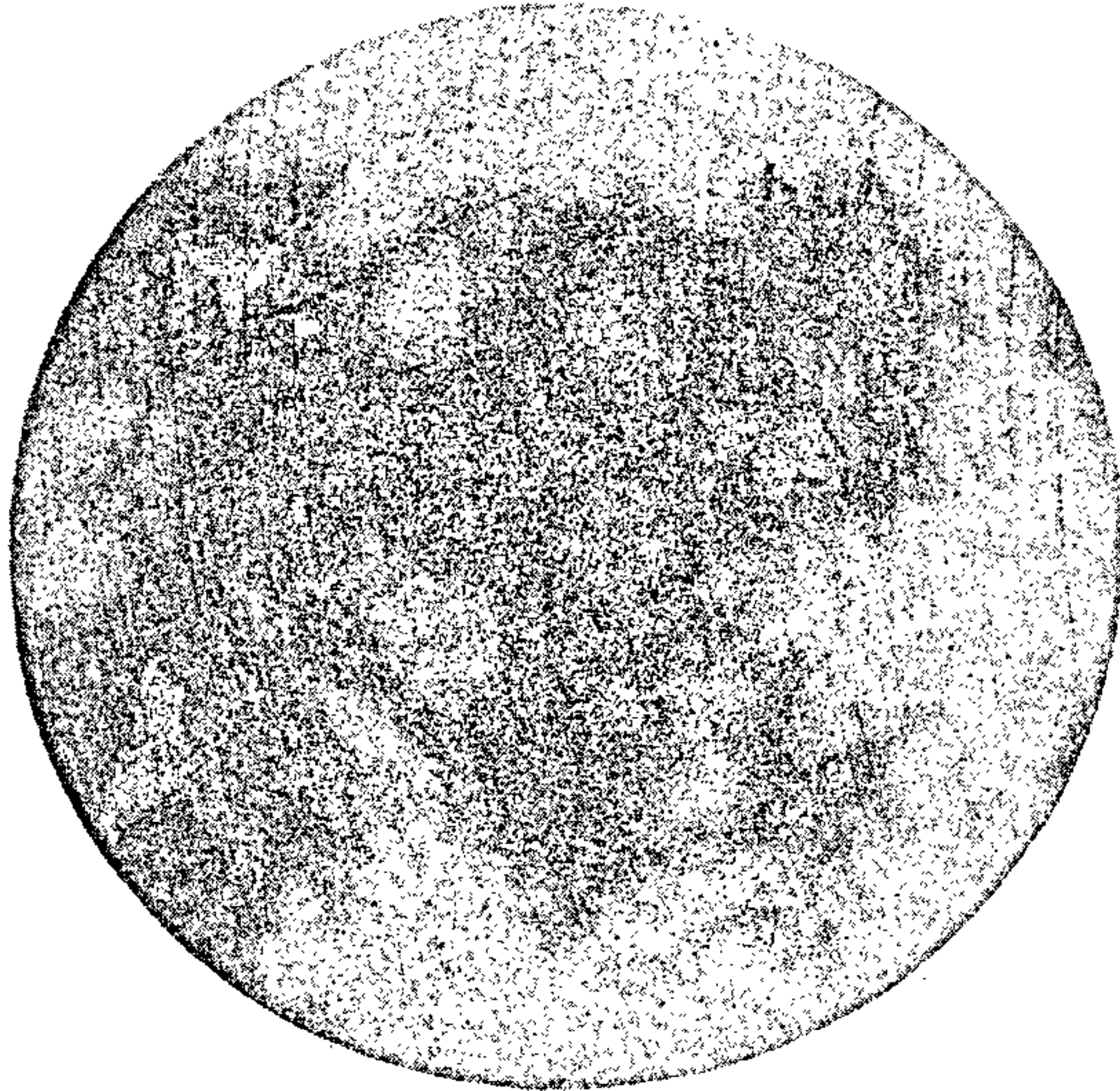
錠型偏析 3 级
