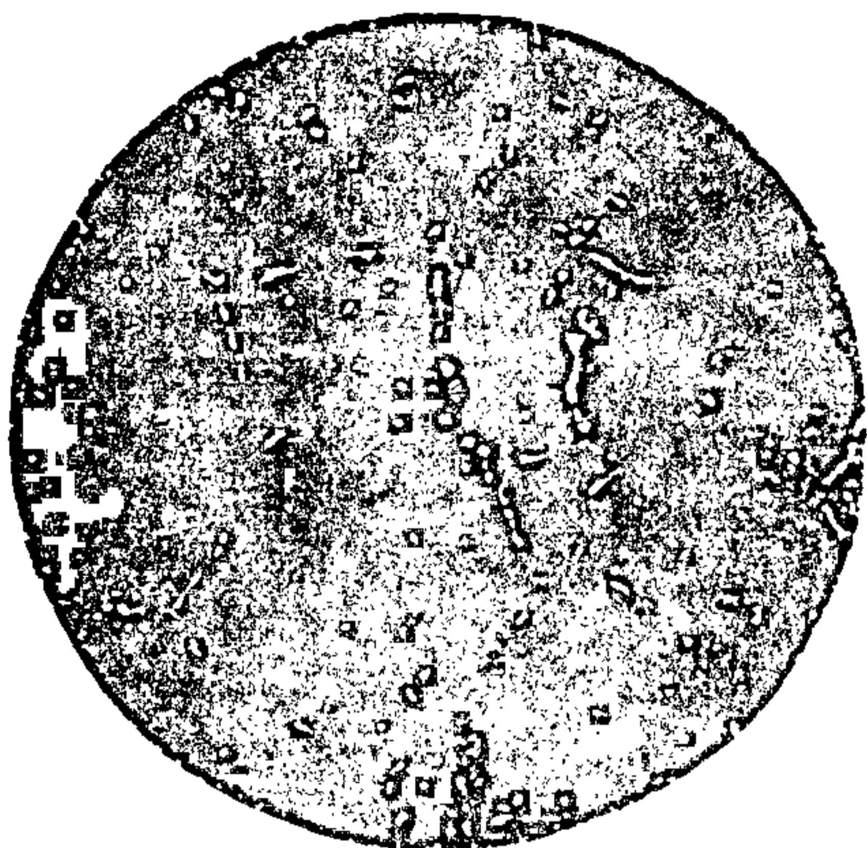
网状碳化物 3级
