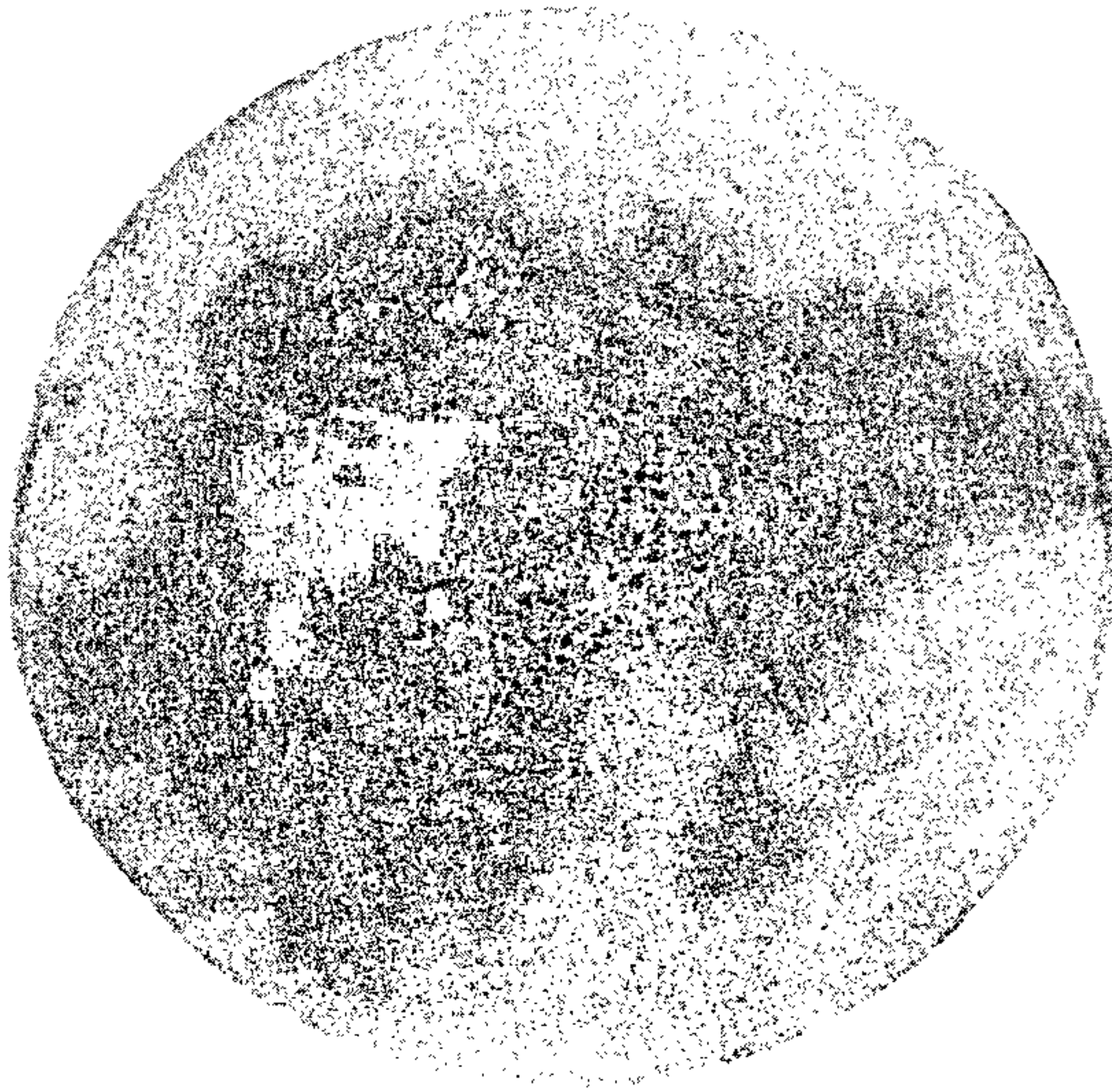
中心疏松 5级
