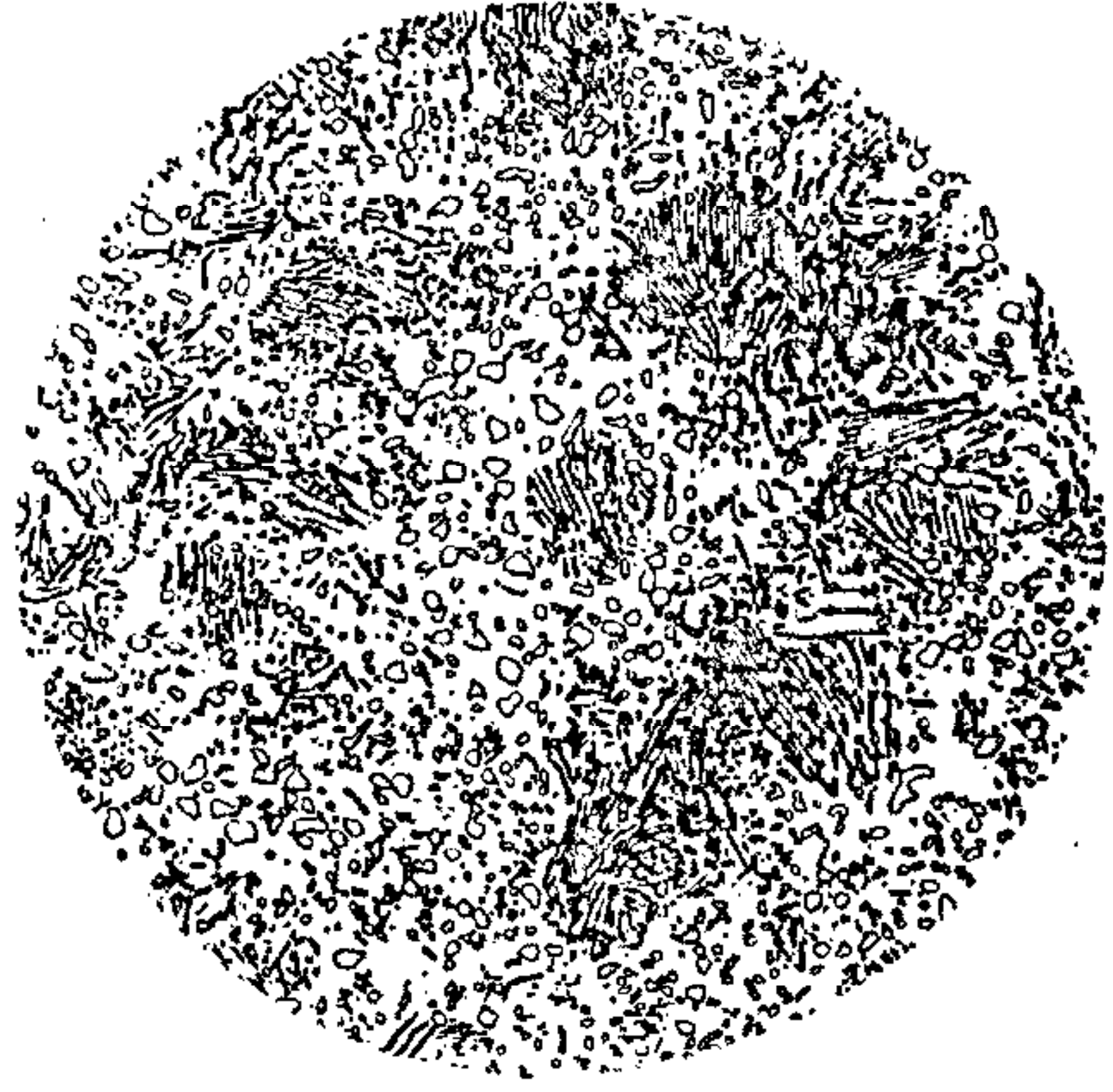
珠光体组织 6级
