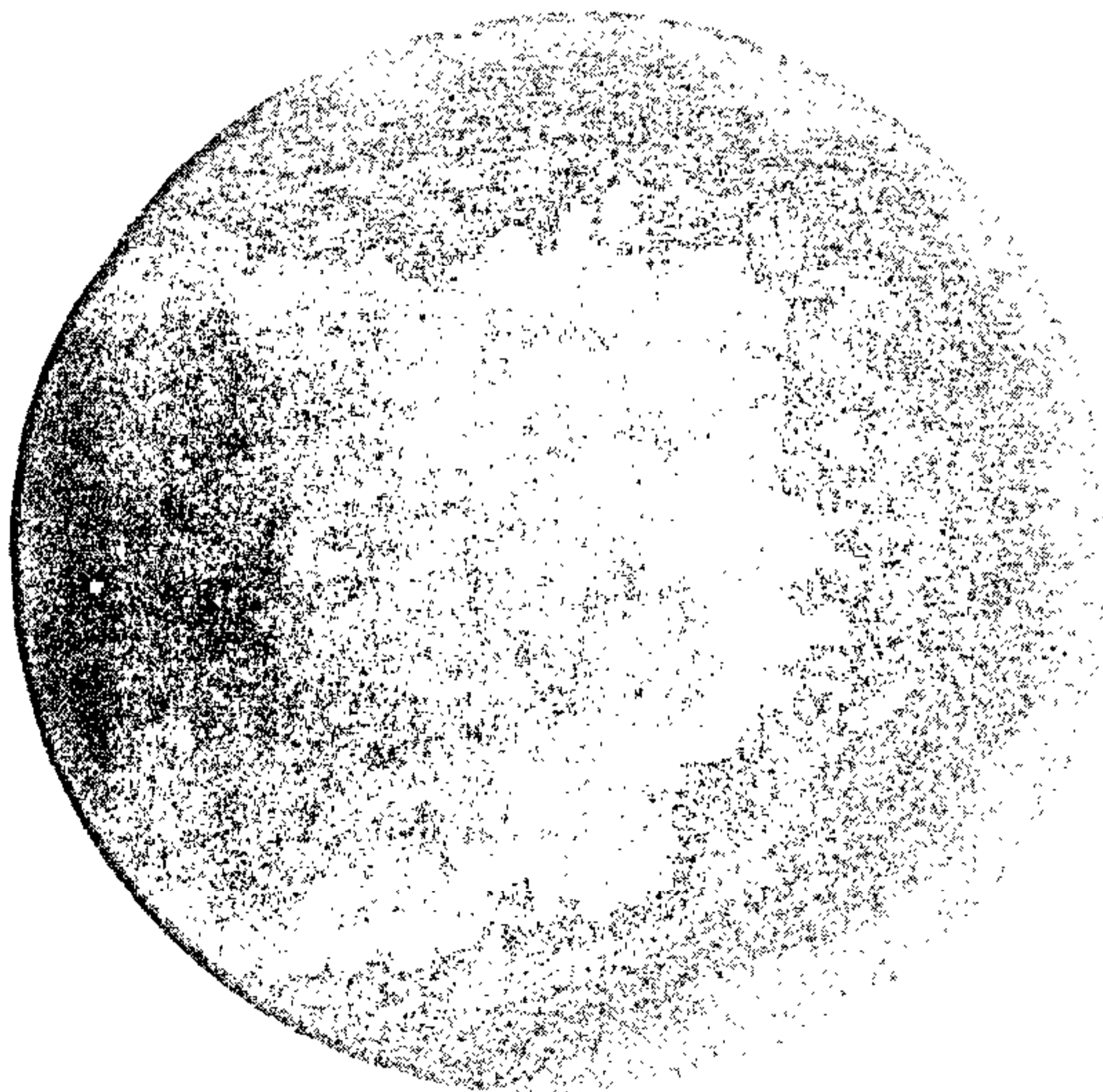
中心疏松 3级
