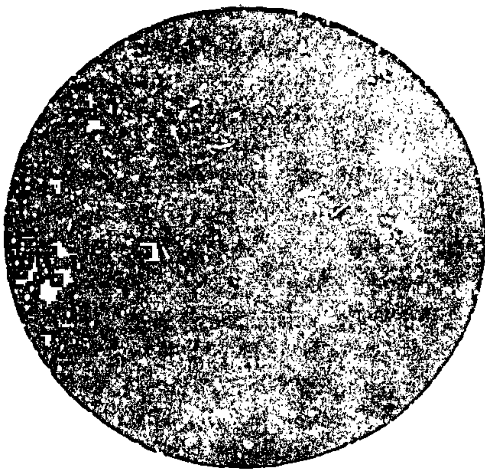
网状碳化物 1级
