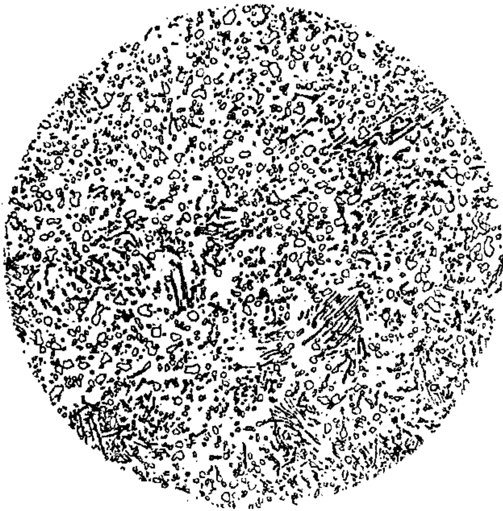
珠光体组织 5级
