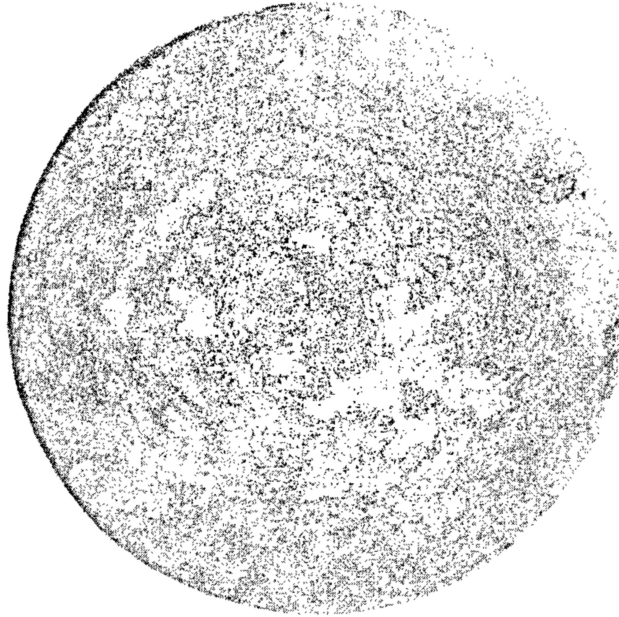
铤型偏析 6级
