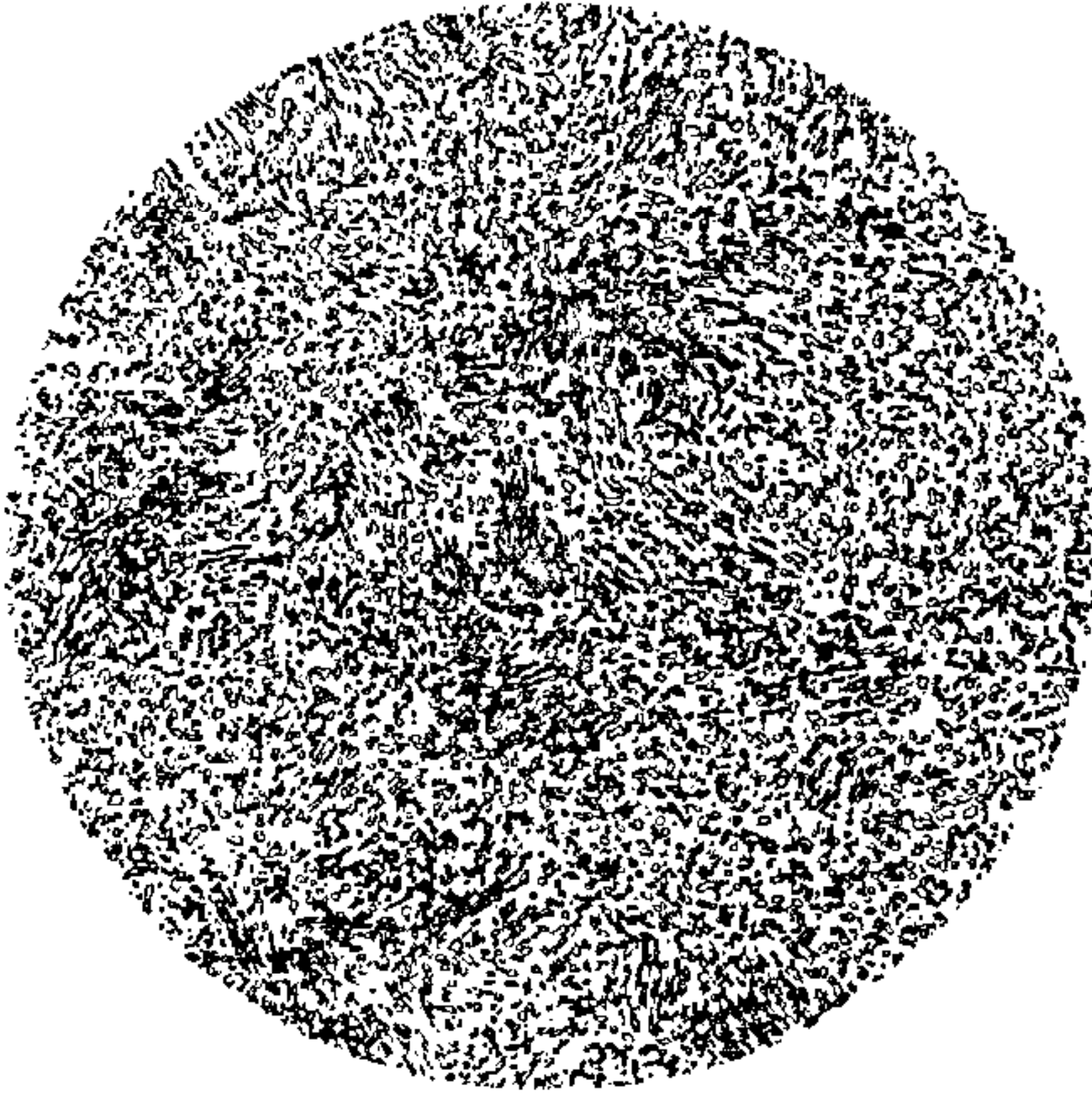
珠光体组织 1级
