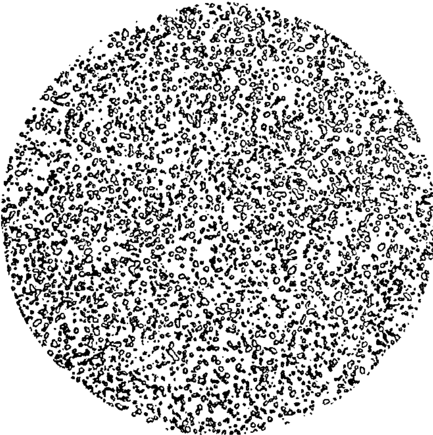
珠光体组织 3级
