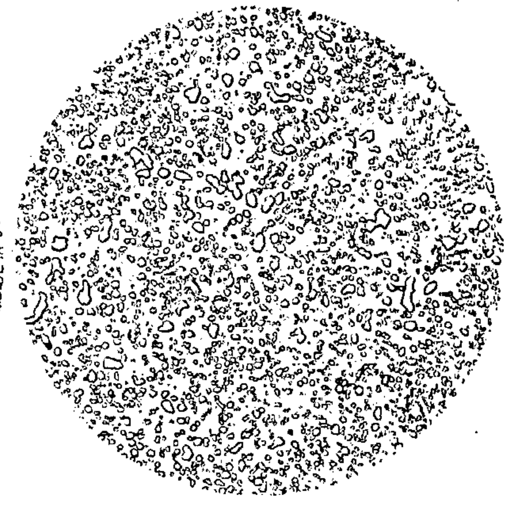
珠光体组织 4级
